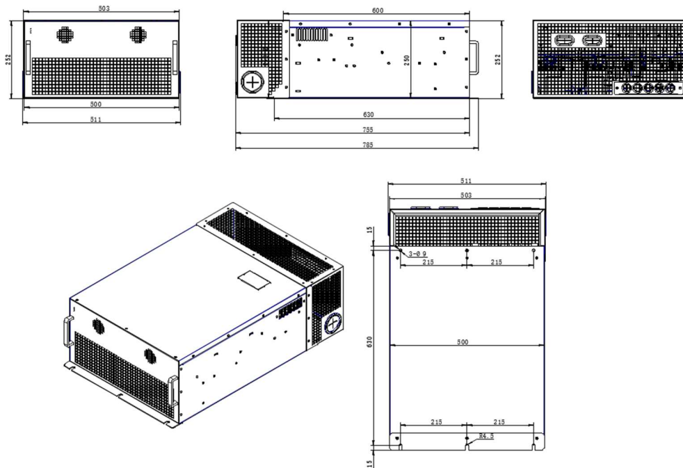
Rysunek 3.7: Wymiary w wykonaniu naściennym model 150kvar 400VAC IP20.
