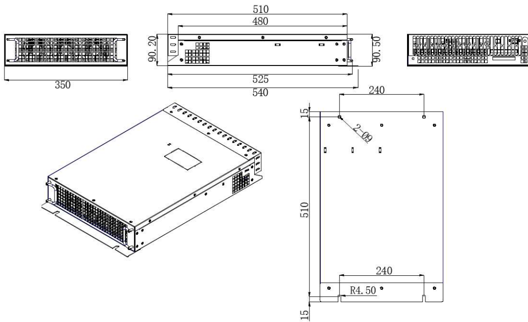
Rysunek 3.2: Wymiary w wykonaniu naściennym CW ASVG model 3-10kvar IP20.
