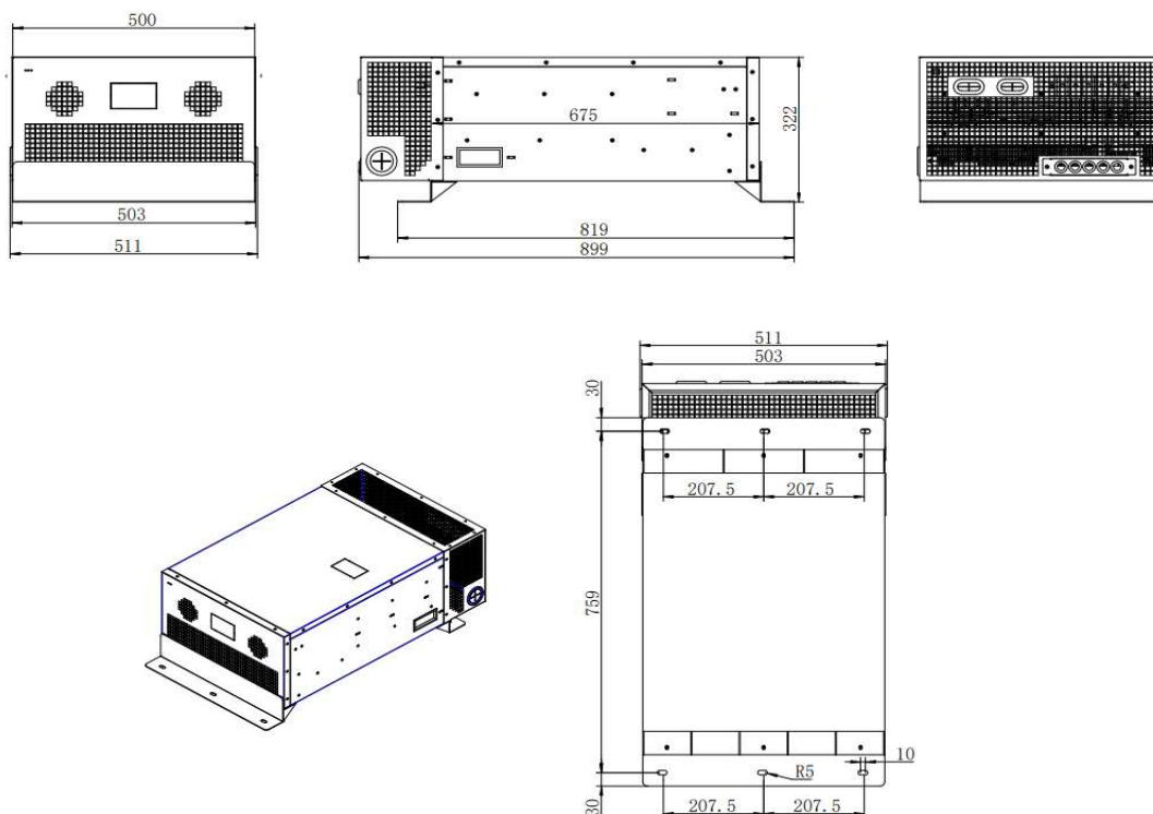
Rysunek 3.8: Wymiary w wykonaniu naściennym model 150kvar 800VAC IP20.
