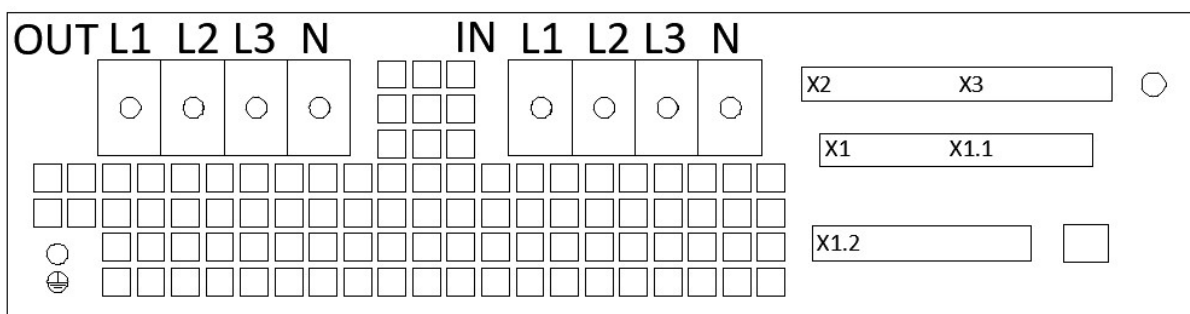
Rysunek 5.4.7: Zaciski przyłączeniowe ASVG-5 kvar.
