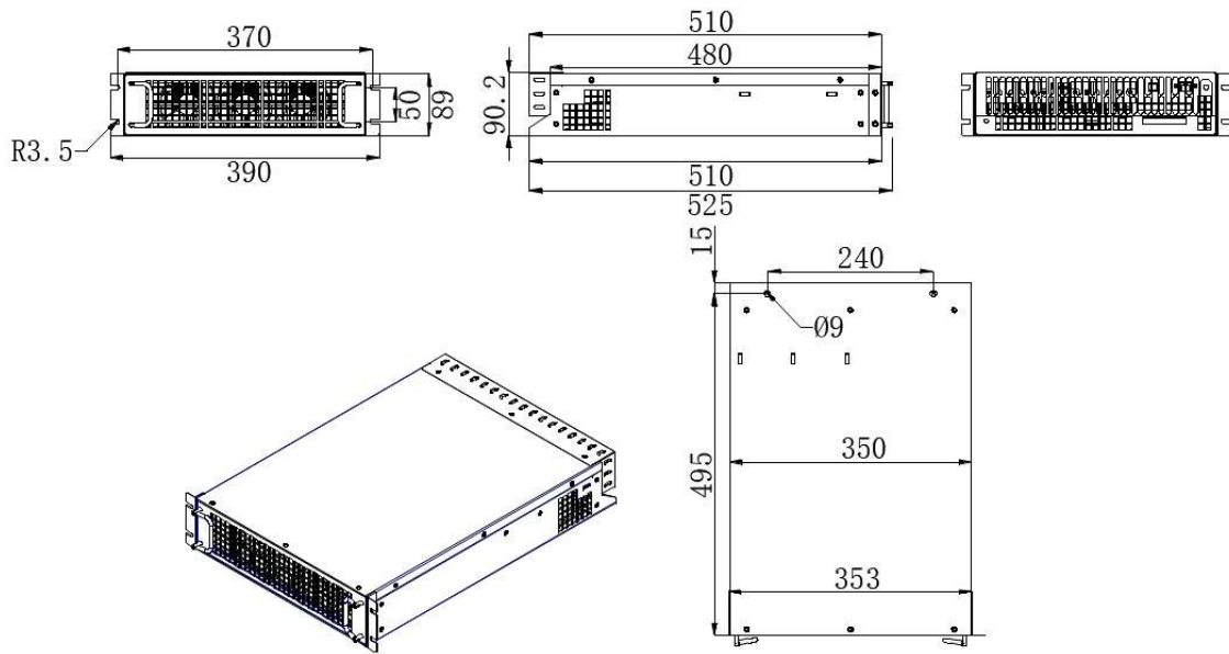
Rysunek 3.7: Wymiary w wykonaniu kompakt rakowym model CR ASVG 3-10kvar IP20.
