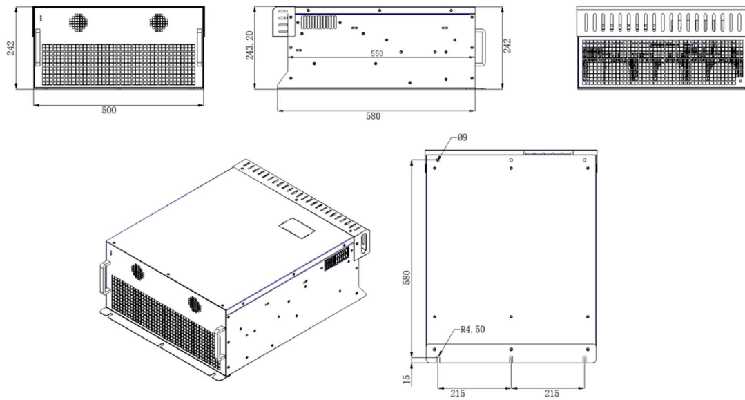
Rysunek 3.6: Wymiary w wykonaniu naściennym modele 75 i 100kvar IP20.
