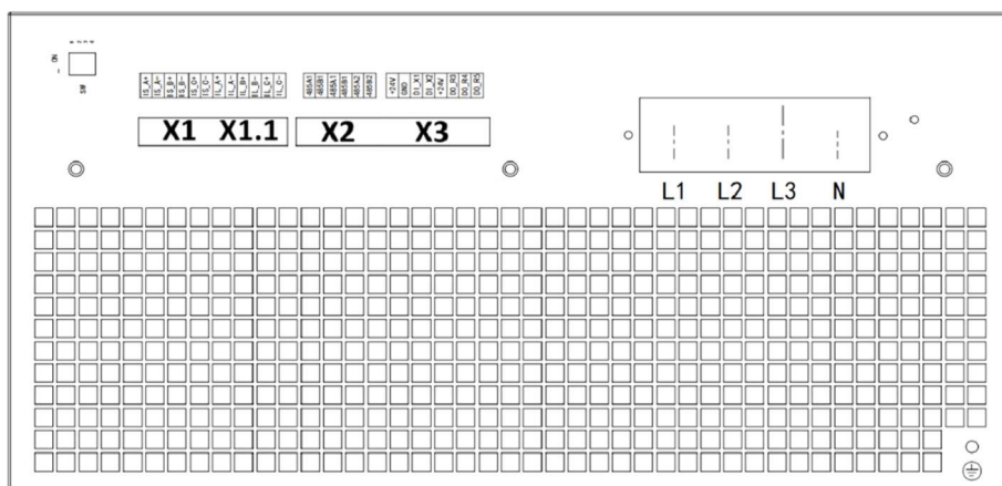
Rysunek 5.4.5: Zaciski przyłączeniowe SVG 50 kvar.
