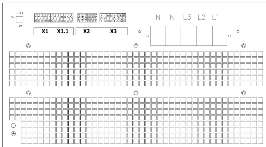
Rysunek 5.4.2: Zaciski przyłączeniowe ASVG 150kvar 800V.
