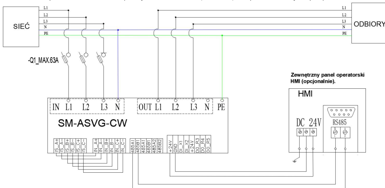
Rysunek 5.7.1 Schemat podłączenia ASVG CW (3-10kvar) z użyciem wewnętrznych przekładników.
