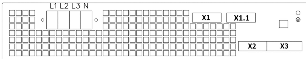
Rysunek 5.4.6: Zaciski przyłączeniowe SVG 10, 15, 20, 35 kvar.
