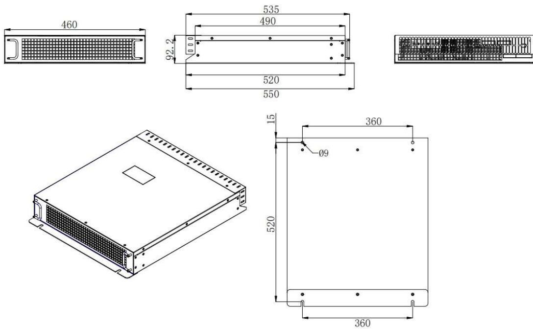
Rysunek 3.3: Wymiary w wykonaniu naściennym modelem 10-35kvar IP20.
