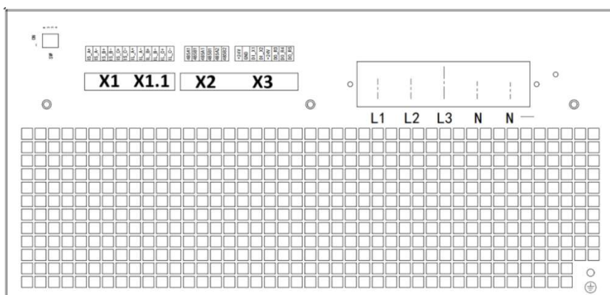
Rysunek 5.4.4: Zaciski przyłączeniowe SVG 75 i 100 kvar.
