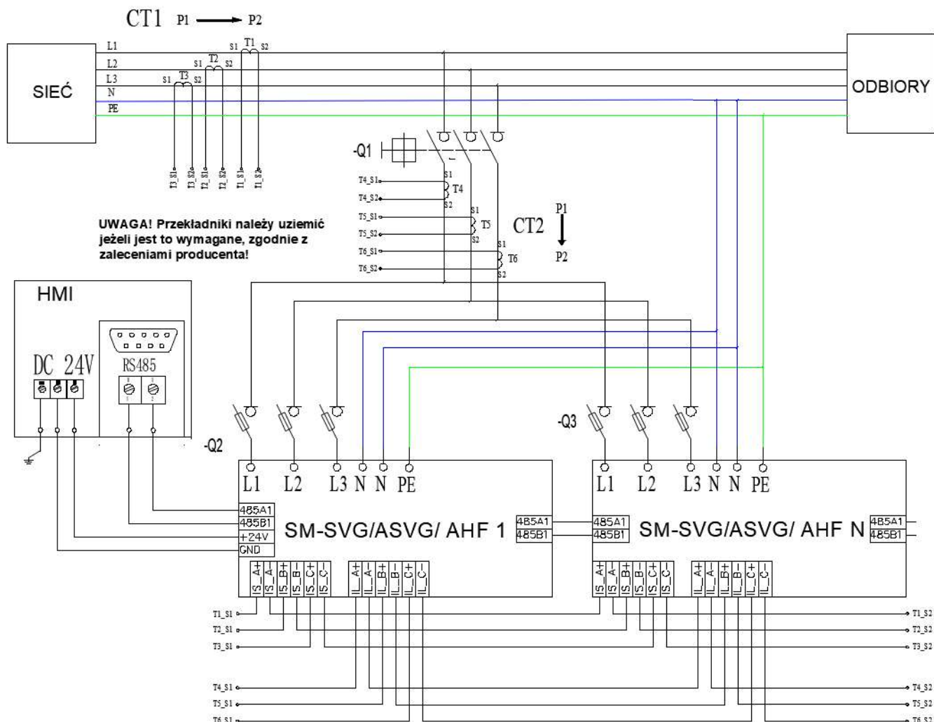
Rysunek 5.6.1: Schemat podłączenie modułów do pracy równoległej SVG(ASVG) w wersji wall i rack.
