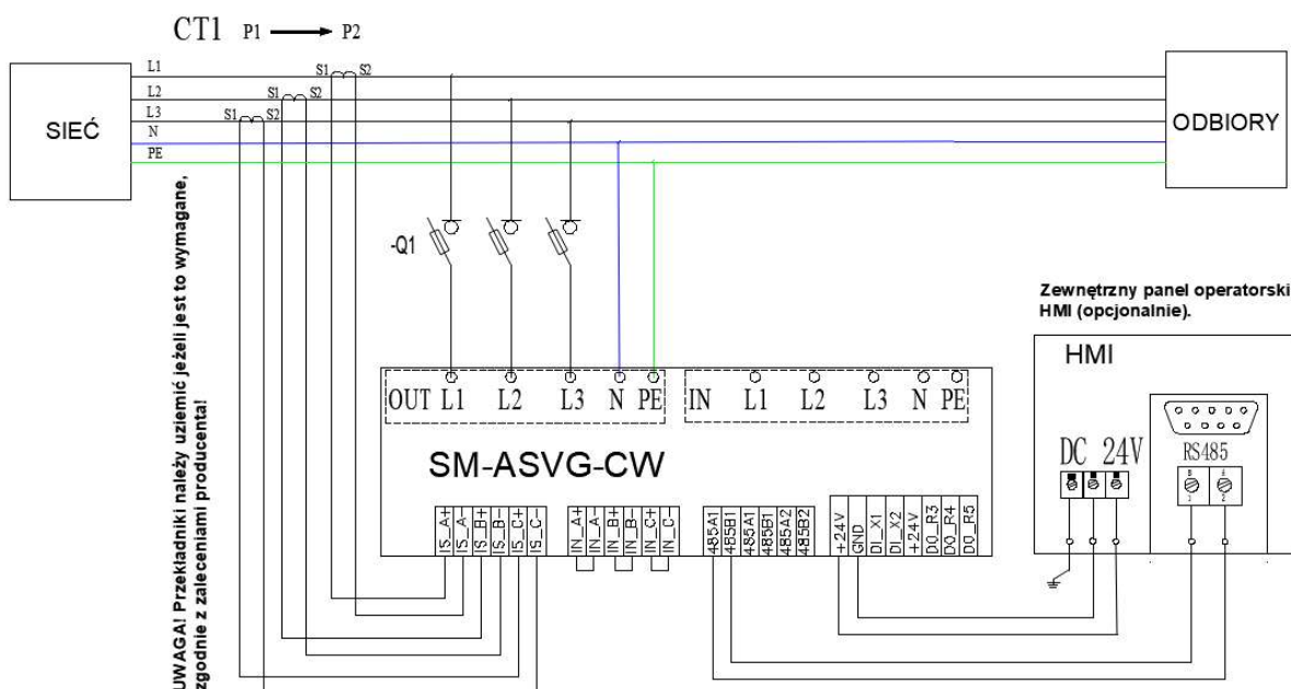
Rysunek 5.8.1 Schemat podłączenia ASVG CW (5-10kvar) z użyciem zewnętrznych przekładników.
