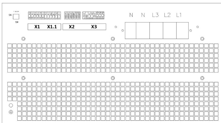
Rysunek 5.4.3: Zaciski przyłączeniowe ASVG 150kvar 800V.
