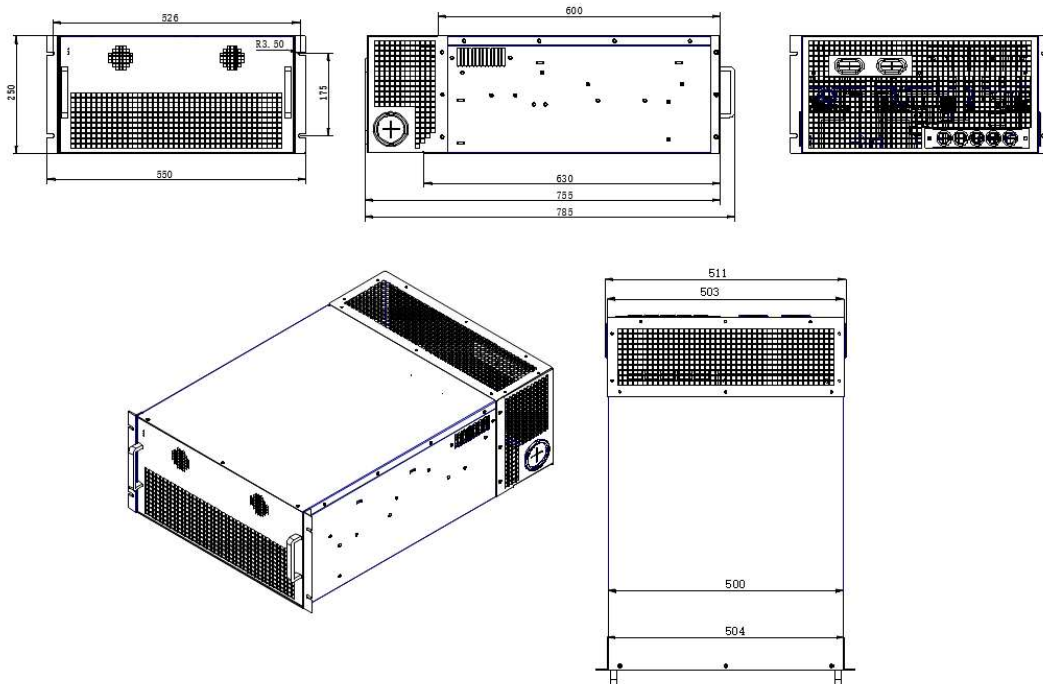
Rysunek 3.11: Wymiary w wykonaniu rakowym model 150kvar 400VAC IP20.
