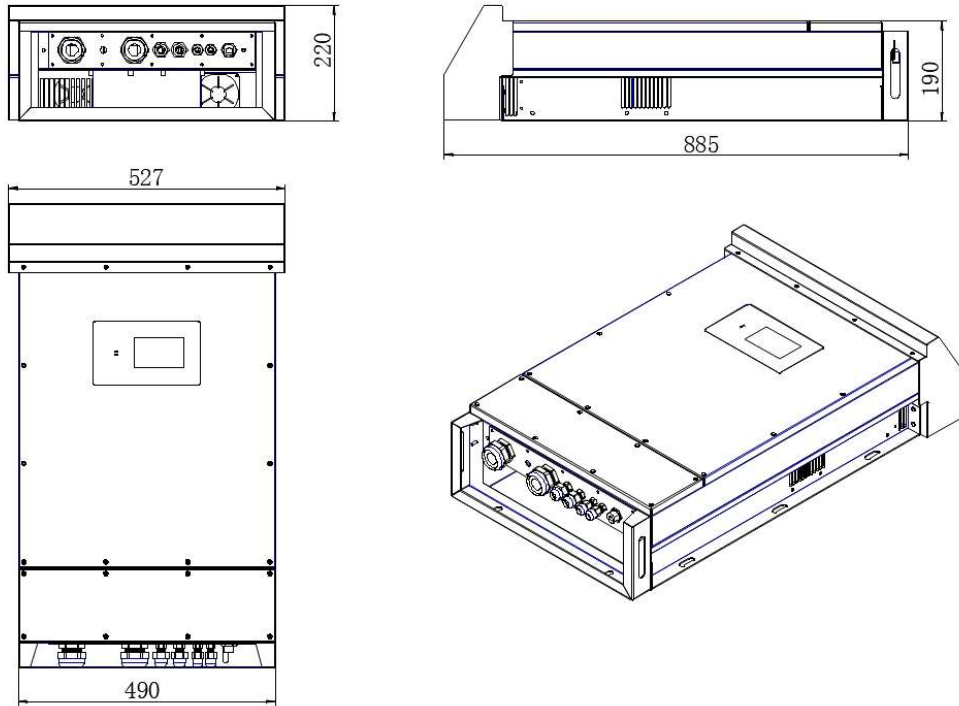
Rysunek 3.4: Wymiary w wykonaniu zewnętrznym IP66.
