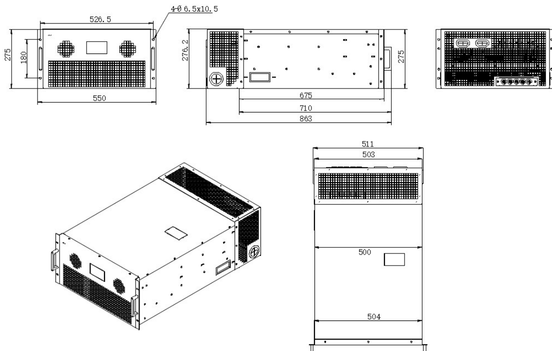
Rysunek 3.12: Wymiary w wykonaniu rakowym model 150kvar 800VAC IP20.
