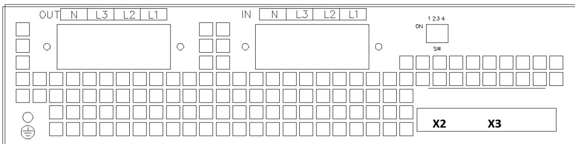
Rysunek 5.4.8: Zaciski przyłączeniowe ASVG-3 kvar.
