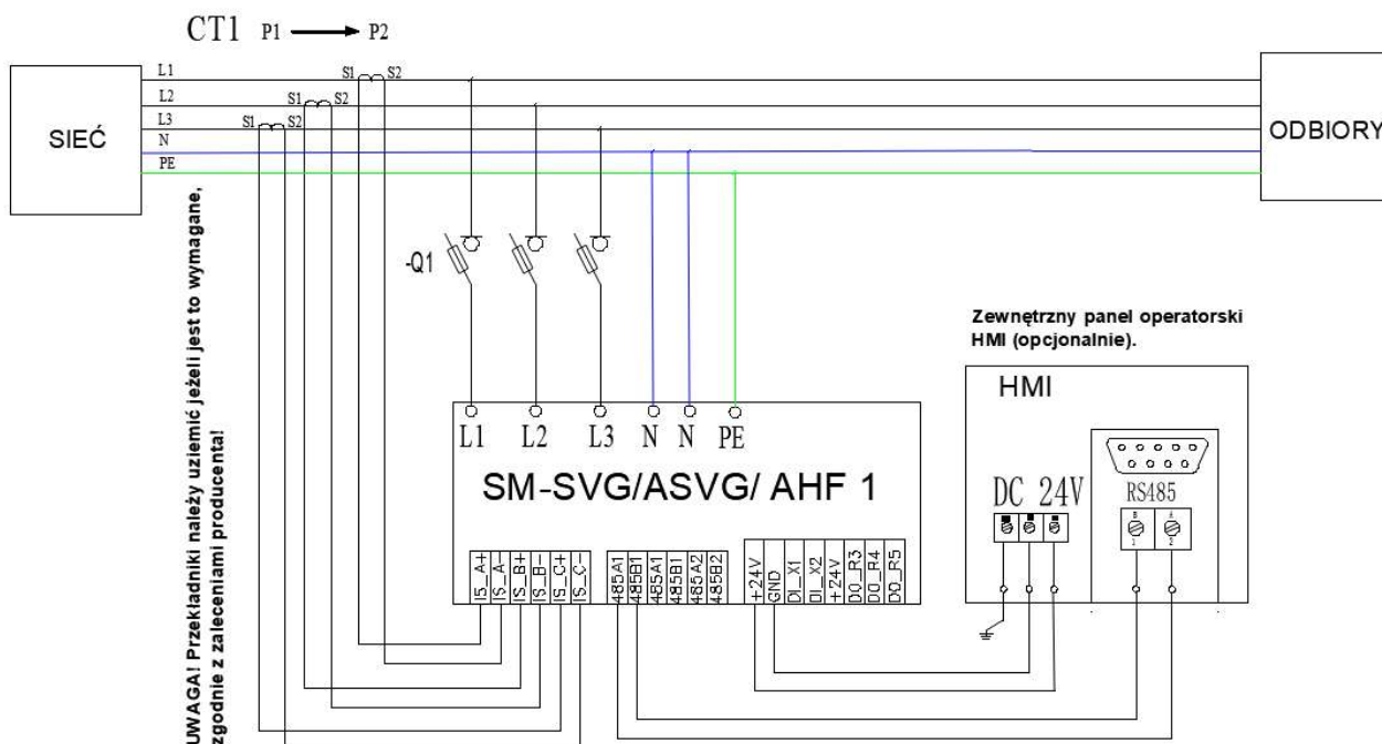
Rysunek 5.5.1: Schemat podłączenie pojedynczego modułu SVG(ASVG) w wersji wall i rack.
